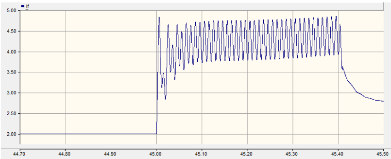
Рис.3. График тока возбуждения для первого эксперимента
