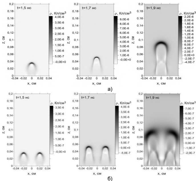
Рис. 1. Изменение во времени t расчётных распределений плотности объёмного заряда \rho в координатной плоскости xOz : а – в одиночном стримере, б – в стримерах, распространяющихся параллельно друг другу при \Delta x_1=0,04 см
