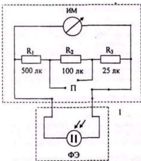
Рис. Устройство люксметра Ю-16
