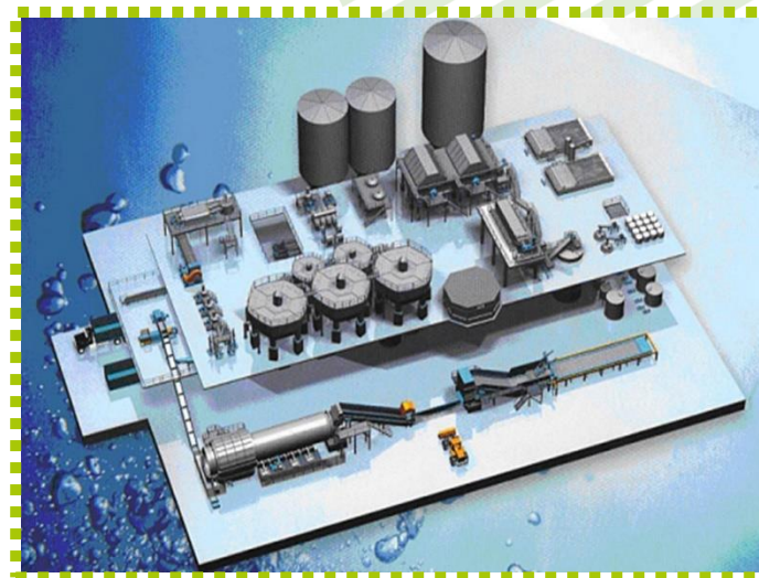
Модель макулатурной линии
